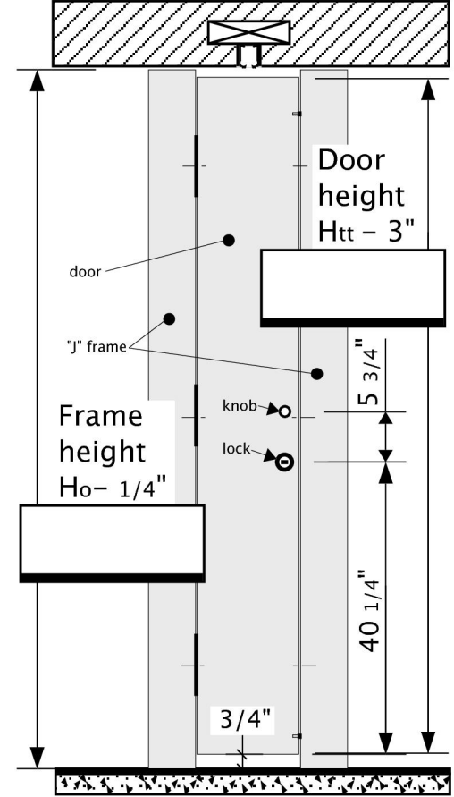
DOOR ELEVATION
